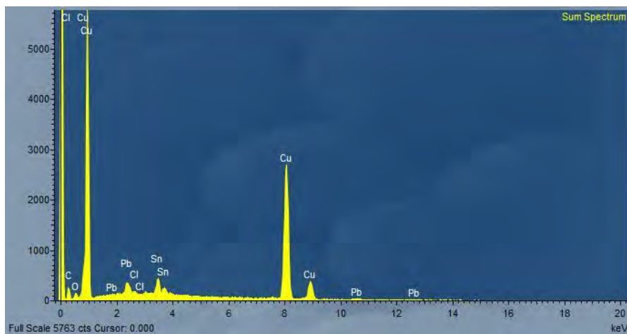
8b. kép – A kibukkanó üde fémrészletek jellemző energiadiszperzív spektruma (C” jelű félgomb) (Cu >> Sn, Pb >> As, Cl, S)
