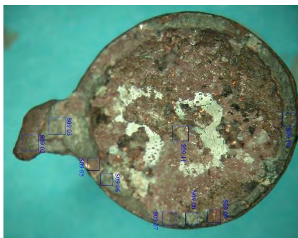
10. kép – Az elemösszetétel meghatározás elektron-mikroszondás vizsgálati helyei („A” jelű félgomb)
