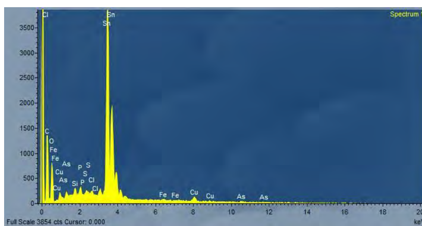
11b. kép – A szürke rétegre jellemző energiadiszperzív spektruma („A” jelű félgomb) ( \text{Sn} \gg \text{Cu}, \text{Pb}, \text{As}, \text{S} )
