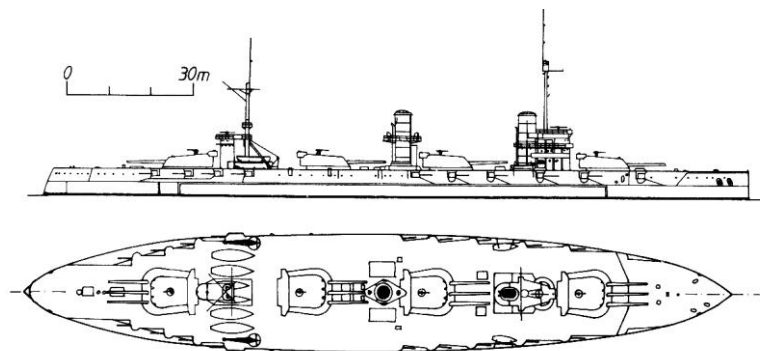
Imperatrice Marija -osztályú csatahajó jobb oldalnézeti és felülnézeti diagrammja. 53
