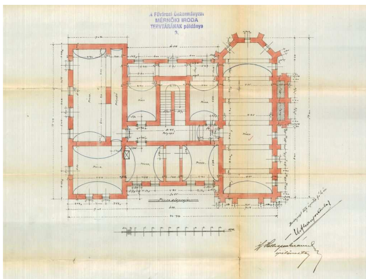
7. A Budapest XI. kerület, Ménesi út 26. szám alatt álló központi ház alaprajza, készítette: Hofhauser Antal (1907. április 4.) 101
