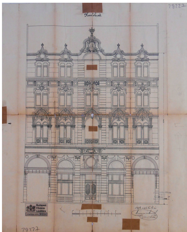
21. Schweiger Gyula, A „Folies Caprice” homlokzatának tervrajza, 1898. (A jelenlegi homlokzat jelentősen átalakított)
