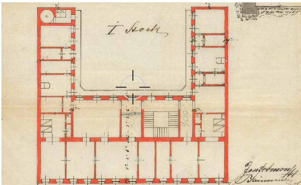
5. Ámon József építész tervrajza (1871) Szentkirályi utca 30. (részlet)
