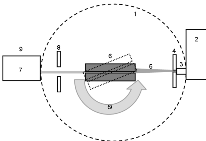
1. ábra A \Theta - 2\Theta röntgen-diffraktométer \Theta=0 paraméterének beállítása, sematikus ábra
