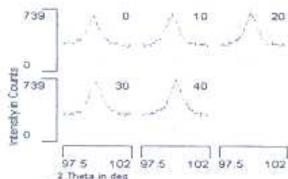
2. ábra a) Raba 3 minta elektrokémiai felületleválasztás után, b) a maradó feszültség méréshez kiválasztott (211) csúcs és a szükséges korrekciók eredménye
