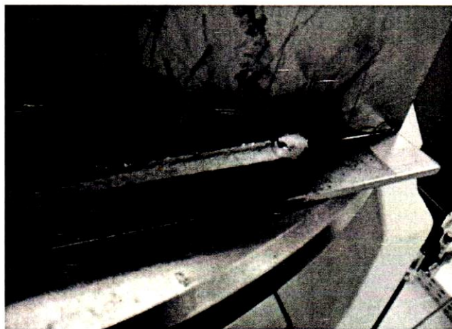
6. ábra. KF-Puls impulzushegesztési eljárással készített sarokvarrat (saját illusztráció).
