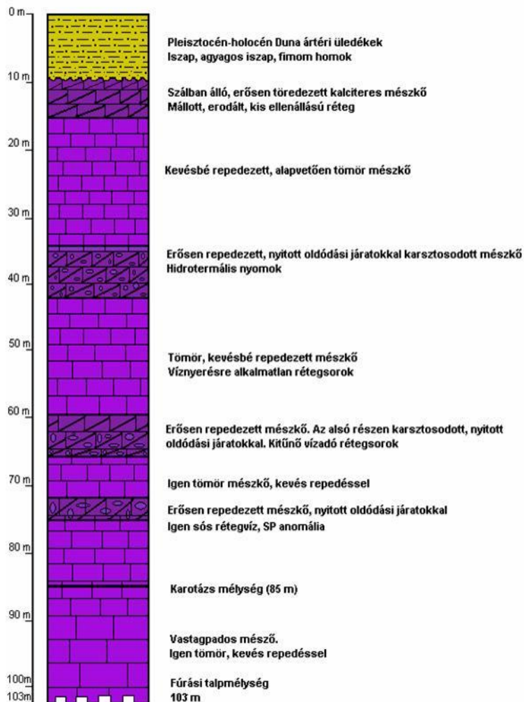
7. ábra: A Vári-pusztá -1. számú vízkutató sekélyfúrás földtani szelvénye
