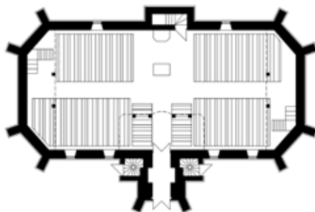
15. kép Magosliget, alaprajz
