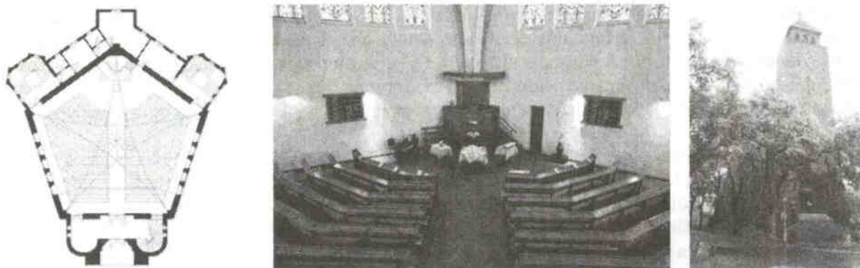
2. ábra. Szeged-Honvéd tér, református templom, alaprajz, belső fotó, külső fotó
