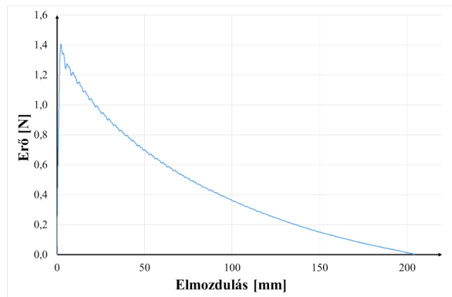
4. ábra Jellegzetes fonalkihúzási görbe
