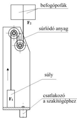
5. ábra A hengeres súrlódásmérés elve
