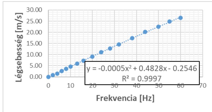
3. ábra: A légcsonnában mért sebességek változó frekvencia mellett
