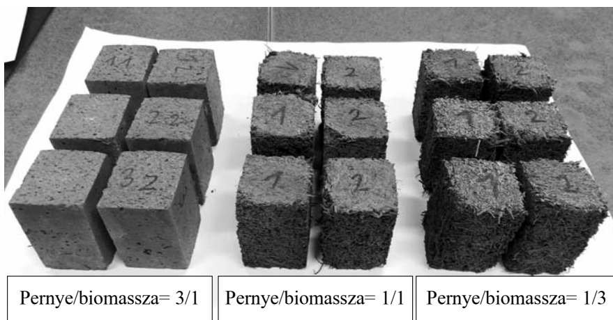
8. ábra: A nyomószilárdság-vizsgálatra előkészített próbatestek
