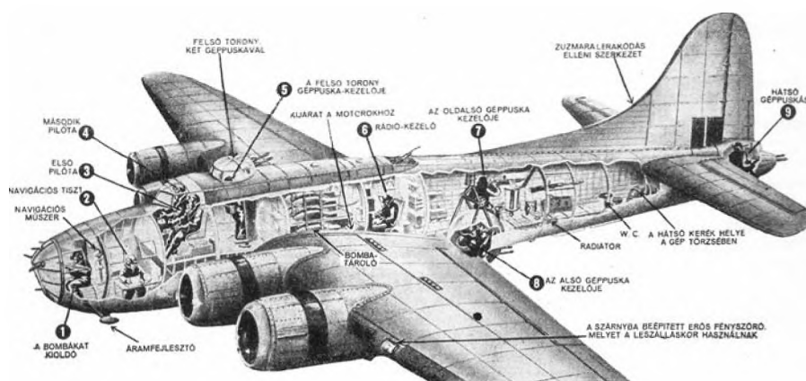
Amerikai B-17-es bombázó, „Flying Fortress” (repülő erőd) felépítése.
