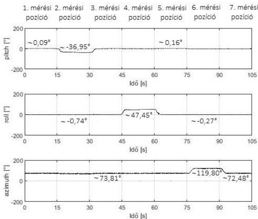
32. ábra: A dőlésmérő kalibráció során megjelenő szögelfordulások mértéke (25. ábra szerinti mérési folyamat)
