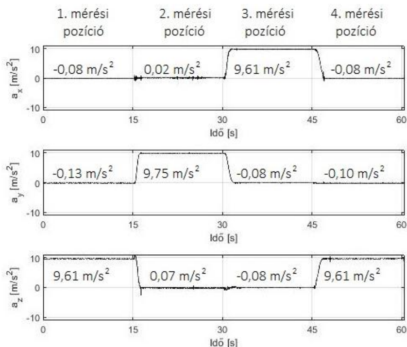
27. ábra A gyorsulásérzékelők kalibrálása során rögzített adatok ( 26. ábra szerinti mérési folyamat)
