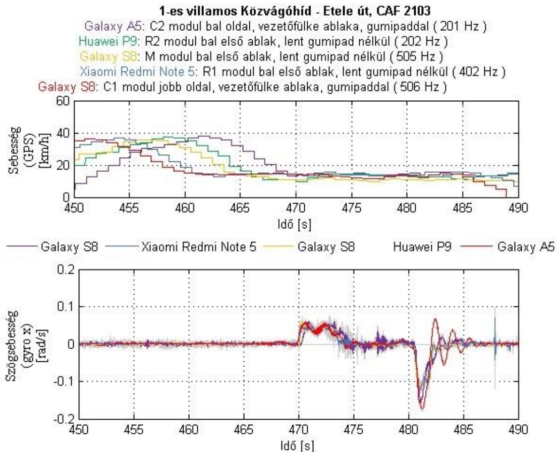
40. ábra: A kocsiszekrény függőleges tengely körüli szögelfordulásának időbeli változása (Etele út / Fehérvári út végállomási szimmetrikusan kifordított kettős vágánykapcsolat, vizsgálat III.)
