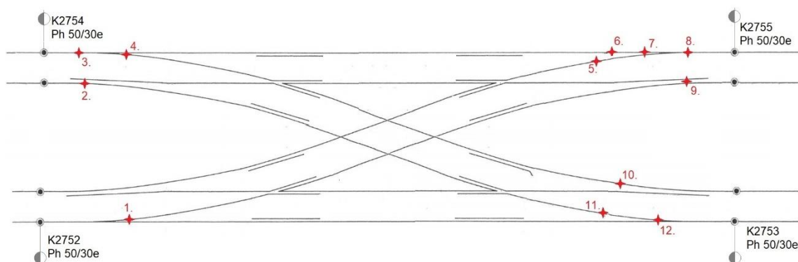
49. ábra: A Savoya Park kettős vágánykapcsolaton észlelt pályahibák [45]
