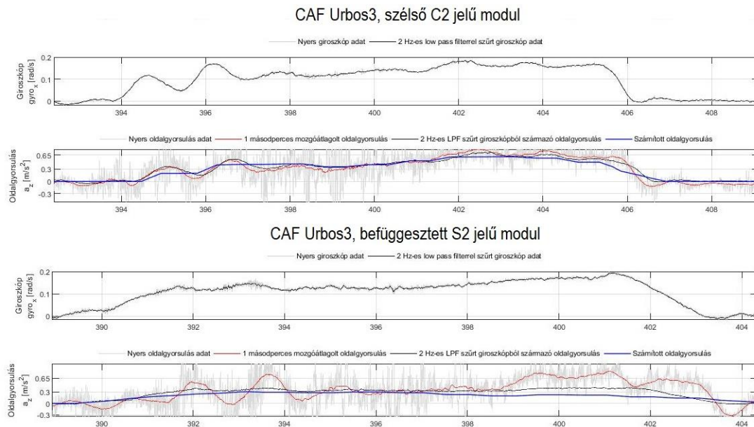
20. ábra: C2 és S2 modulok rögzített mozgásadatai
