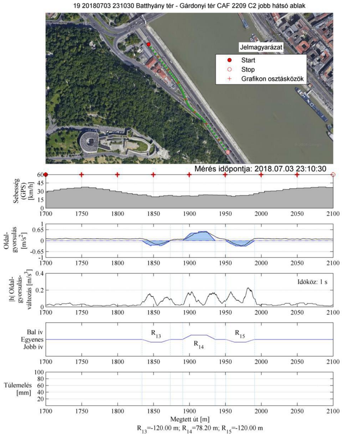
14. ábra: Az okostelefonnal mért oldalgyorsulás adatok összehasonlítása a gyakorlatban széleskörűen alkalmazott közelítő képletekkel (konzulensi segítséggel történő kiértékelés)
