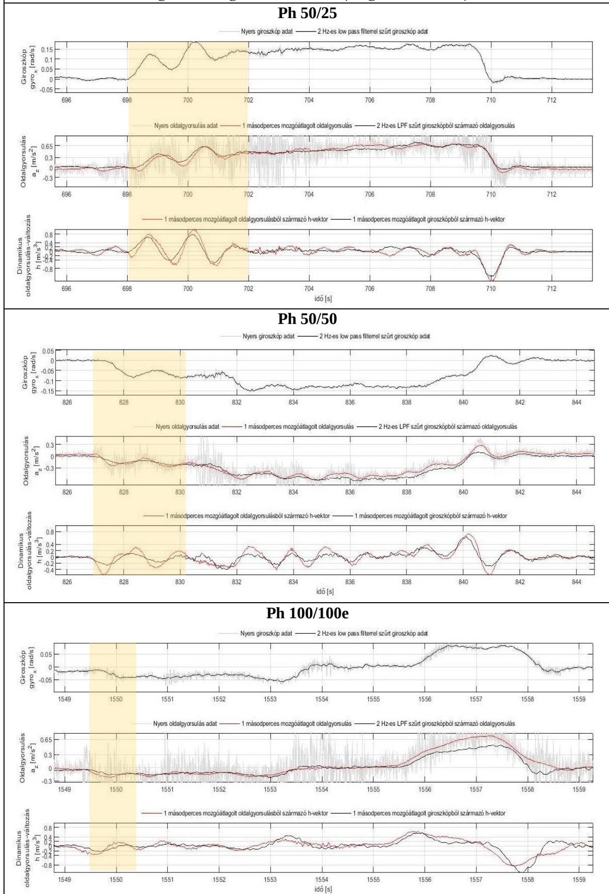
24. ábra: Szabálytalan járműmozgások mértékének összehasonlítása különböző sugarú és végérintő szögű kitérők esetén (sárgával kiemelve)
