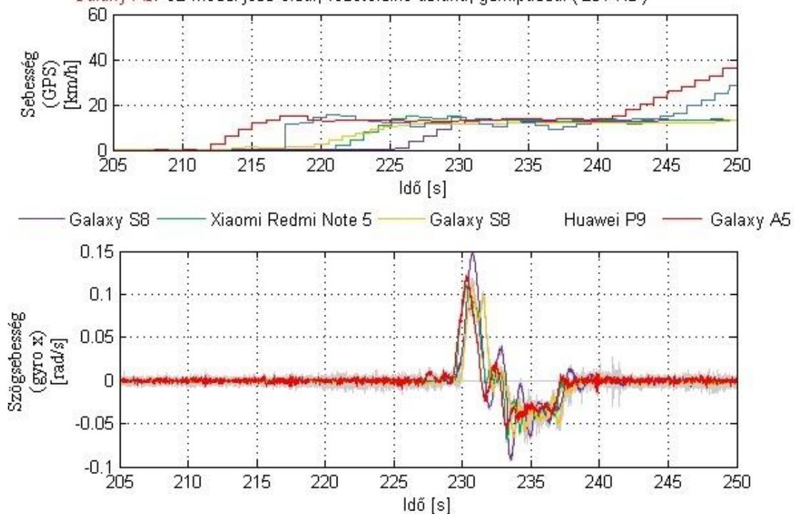
39. ábra: A kocsiszekevény függőleges tengely körüli szögelfordulásának időbeli változása (Etele út/Fehérvári út végállomási szimmetrikusan kifordított kettős vágánykapcsolat, vizsgálat II.)
