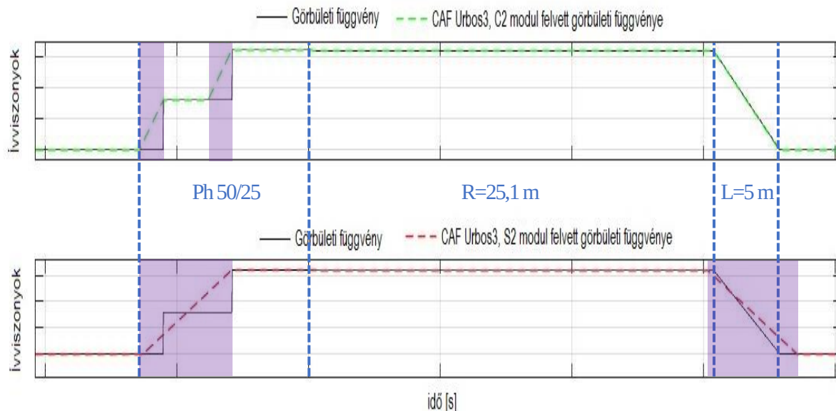
18. ábra: A feltételezett mozgásérzékelő hosszakból adódó görbületi függvények ábrái
