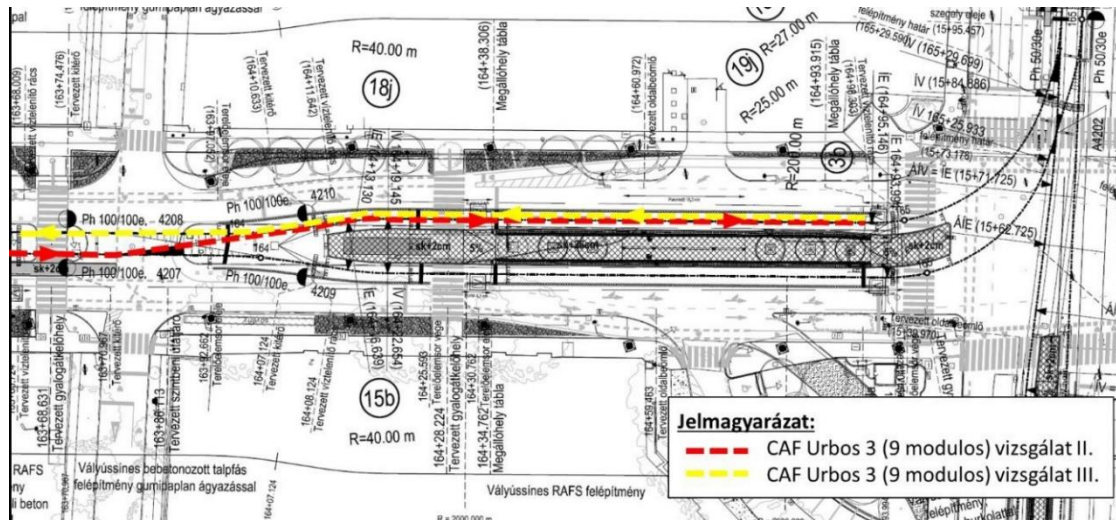
38. ábra: Etele út / Fehérvári úti vágánykapcsolat helyszínrajza a felmért szakaszok és a mérési irányok jelölésével (a mérési menetek részletes kiértékelése és a mérési grafikonok a 42. és a 44. ábrákon tekinthetők meg)
