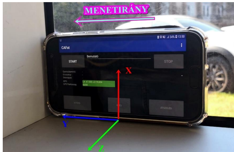
12. ábra: Célszerű mérési elrendezés a CAF villamos ablakának alsó sarkában (gumipaddal rögzítve)
