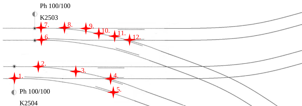
52. ábra: A Döbrentei téri pályaelágazás használatból eredő avulási jelenségeinek elhelyezkedése [45]
