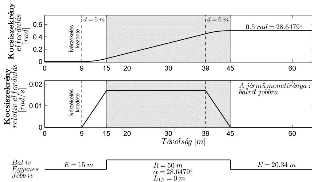
15. ábra: Egy 6 m-es forgócsap távolságú, két forgóvázaz jármű ívrézkélese átmenetiív nélküli ívben (a jármű balról jobbra haladt végig az íven állandó sebességgel (konzulensi segítséggel történő kiértékelés)
