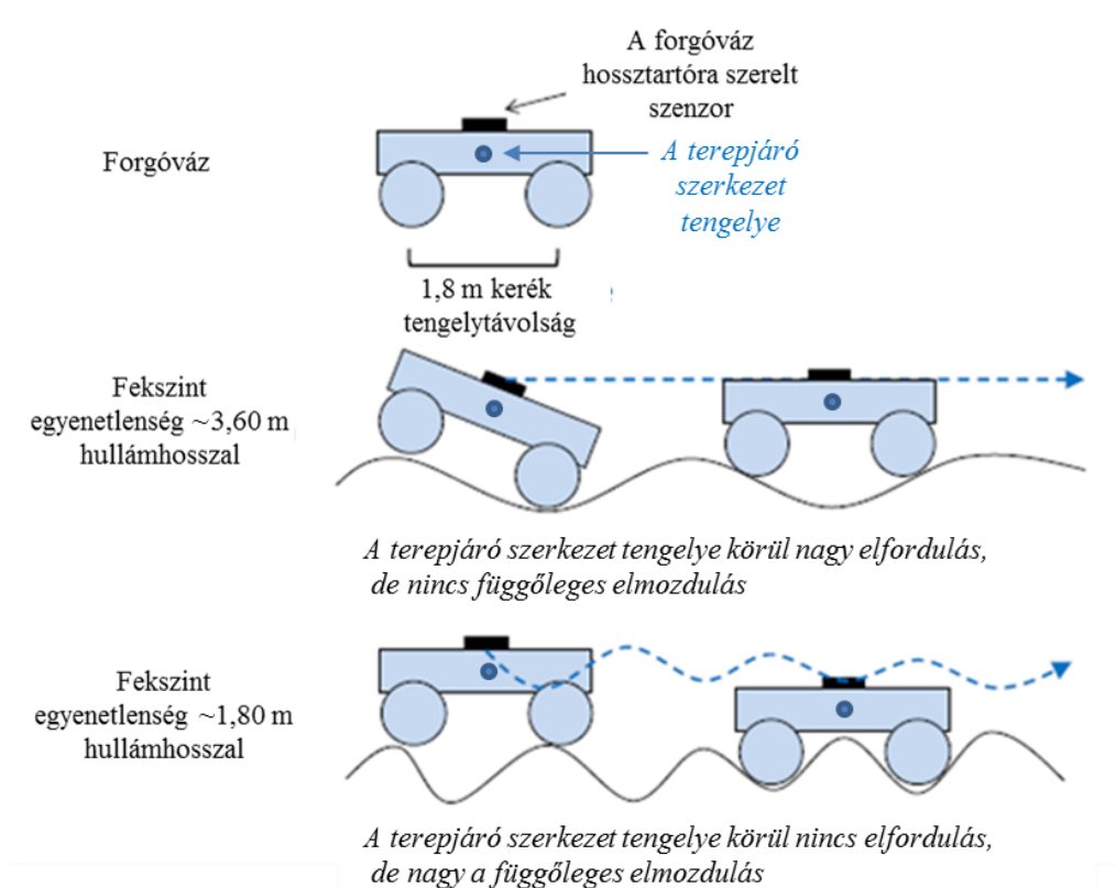
6. ábra: A forgóváz-hossztartóra szerelt szenzor geometriai szűrési effektusa a pályahibák érzékelése szempontjából [18]
