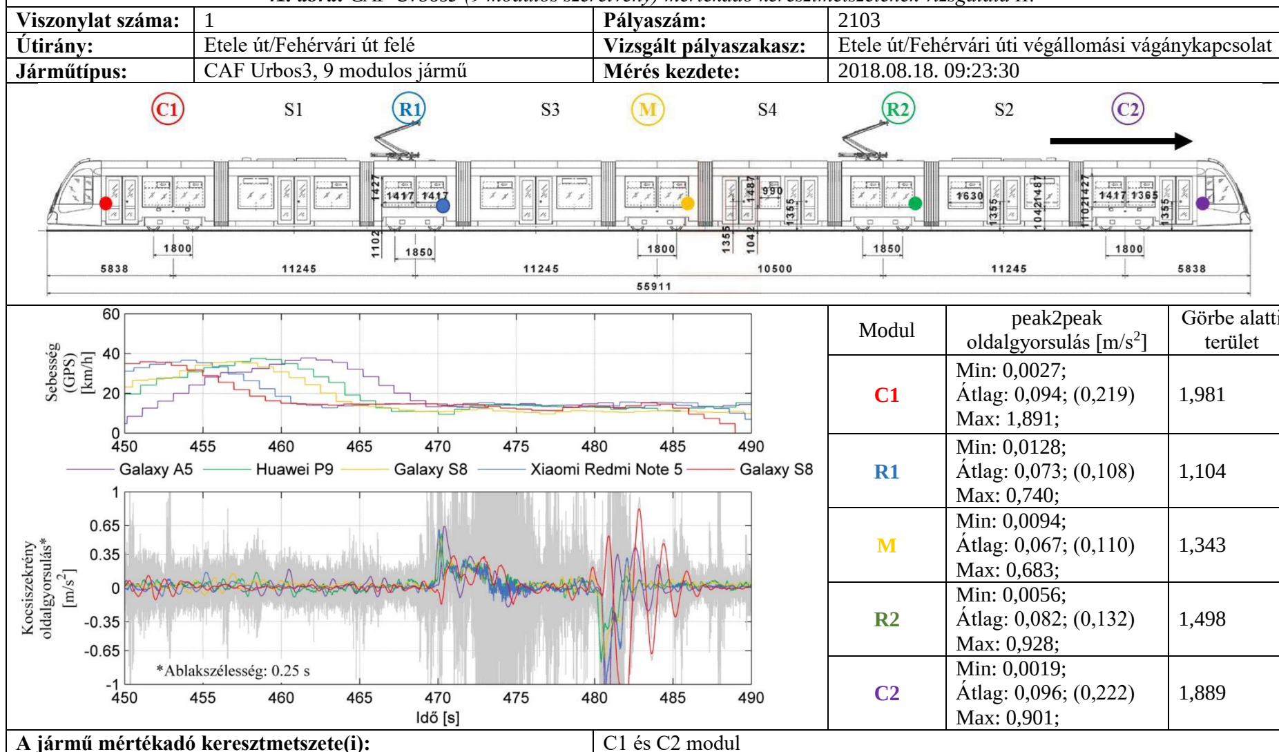
41. ábra: CAF Urbos3 (9 modulος szerelvény) mértékadó keresztmetszetének vizsgálata II.
