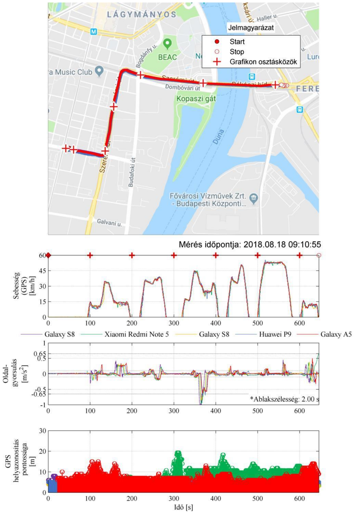
34. ábra: CAF 9 modulok szerelvény vizsgált keresztmetszeteiben rögzített oldalgyorsulás (Etele út/Fehérvári út - Közvágóhíd)
