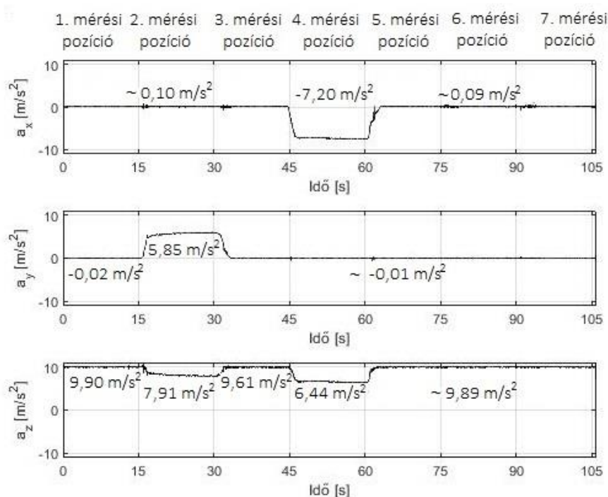
30. ábra: A dőlésmérő szenzor kalibrációjának gyorsulásadatokat tartalmazó grafikonja (29. ábra szerinti mérési folyamat)
