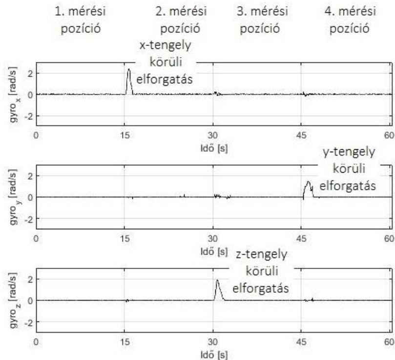
28. ábra: A giroszkóp kalibrálása során rögzített adatok (26. ábra szerinti mérési folyamat)
