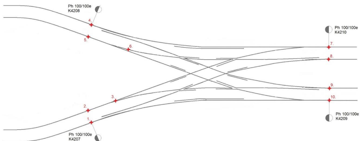
50. ábra: Az Etele út/Fehérvári út végállomás vágánykapcsolatának hibahelyei [45]
