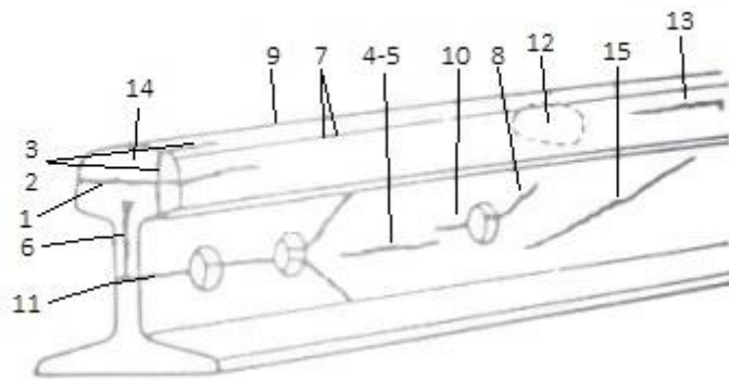
2. ábra: Leggyakrabban előforduló sínhibák 1 Vízszintes fejrepedés a sínvégeken; 2-3 Függőleges és hosszirányú repedés a sínfejen; 4-5 Közel vízszintes repedés a síngerincen; 6 Lunkerosság; 7-8-9-10-11 Furatból kiinduló ferde repedések; 12 Vese alakú törés; 13 Vízszintes alakú fejrepedés; 14 Lemezes leválás a járósíkon; 15 Hegesztések hibái [6]
