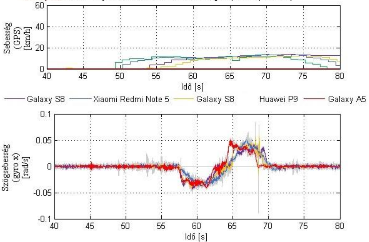
46. ábra: A kocsiszekrény függőleges tengely körüli szögelfordulásának időbeli változása (Batthyány tér vonali visszafogás; CAF 2209, 5 modulos szerelvény)
