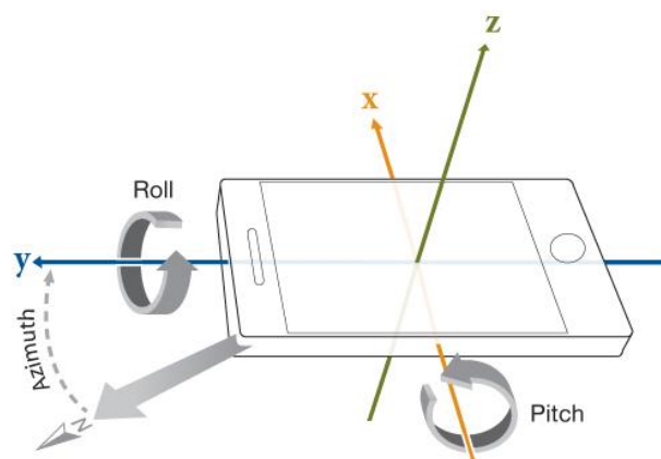
11. ábra: A szenzorok mérési tengelyeinek és a pozitív forgási irányok értelmezése [40]
