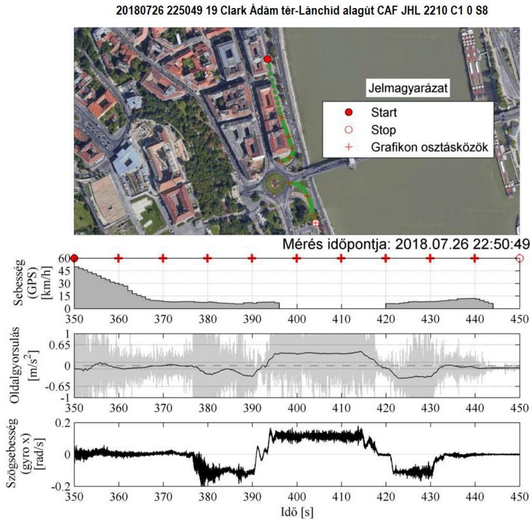
16. ábra: Ívek kimutatása gyorsulás és giroszkóp adatokkal (CAF villamossal - Samsung Galaxy S8 készülékkel, konzulensi segítséggel történő kiértékelés)
