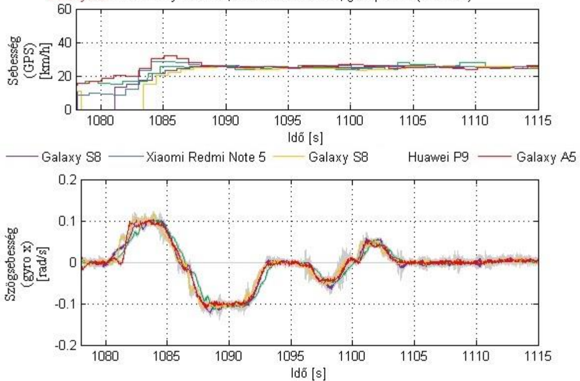
45. ábra: A kocsiszekrény függőleges tengely körüli szögelfordulásának időbeli változása (Margit híd, fonódó pályaszakasz, CAF 2209, 5 modulos szerelvény)
