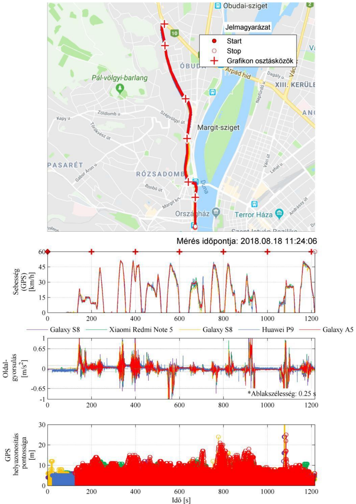
43. ábra: CAF (5 modulos) vizsgált keresztmetszeteiben rögzített oldalgyorsulás (Bécsi út/Vörösvári út - Batthyány tér)
