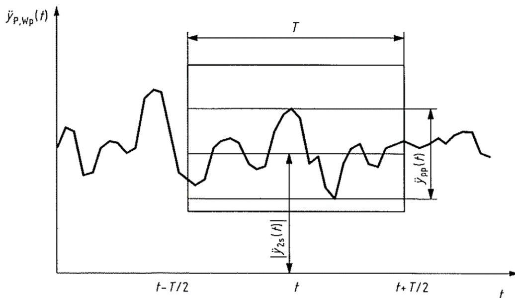
8. ábra: P_{DE} komfortjellemző számításának alapelve [39]
