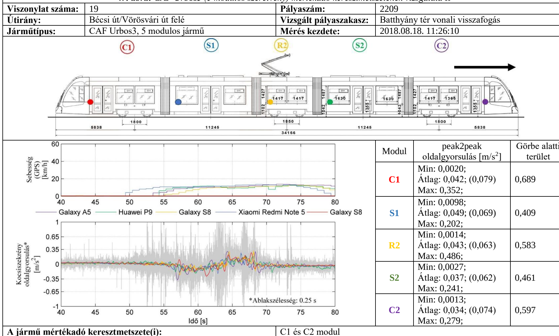
47. ábra: CAF Urbos3 (5 modulος szerelvény) mértékadó keresztmetszetének vizsgálata II
