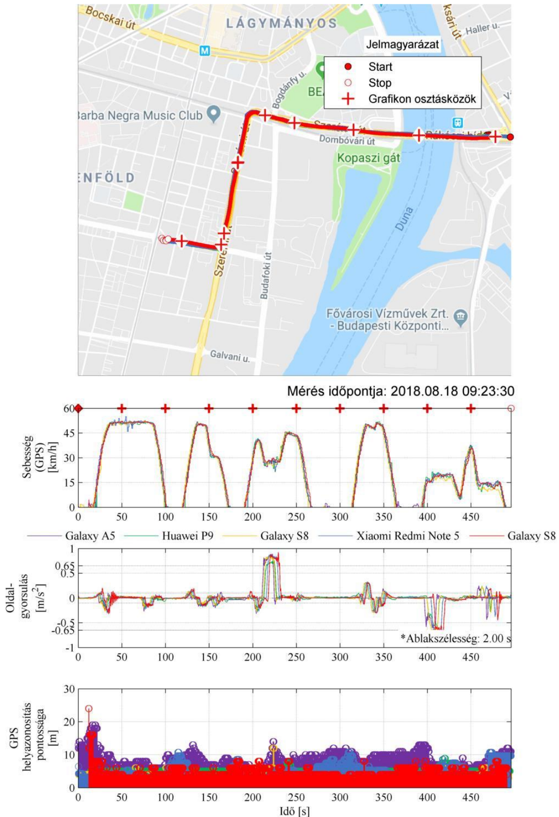
35. ábra: CAF 9 modulós szerelvény vizsgált keresztmetszeteiben rögzített oldalgyorsulás (Közvágóhíd - Etele út/Fehérvári út)
