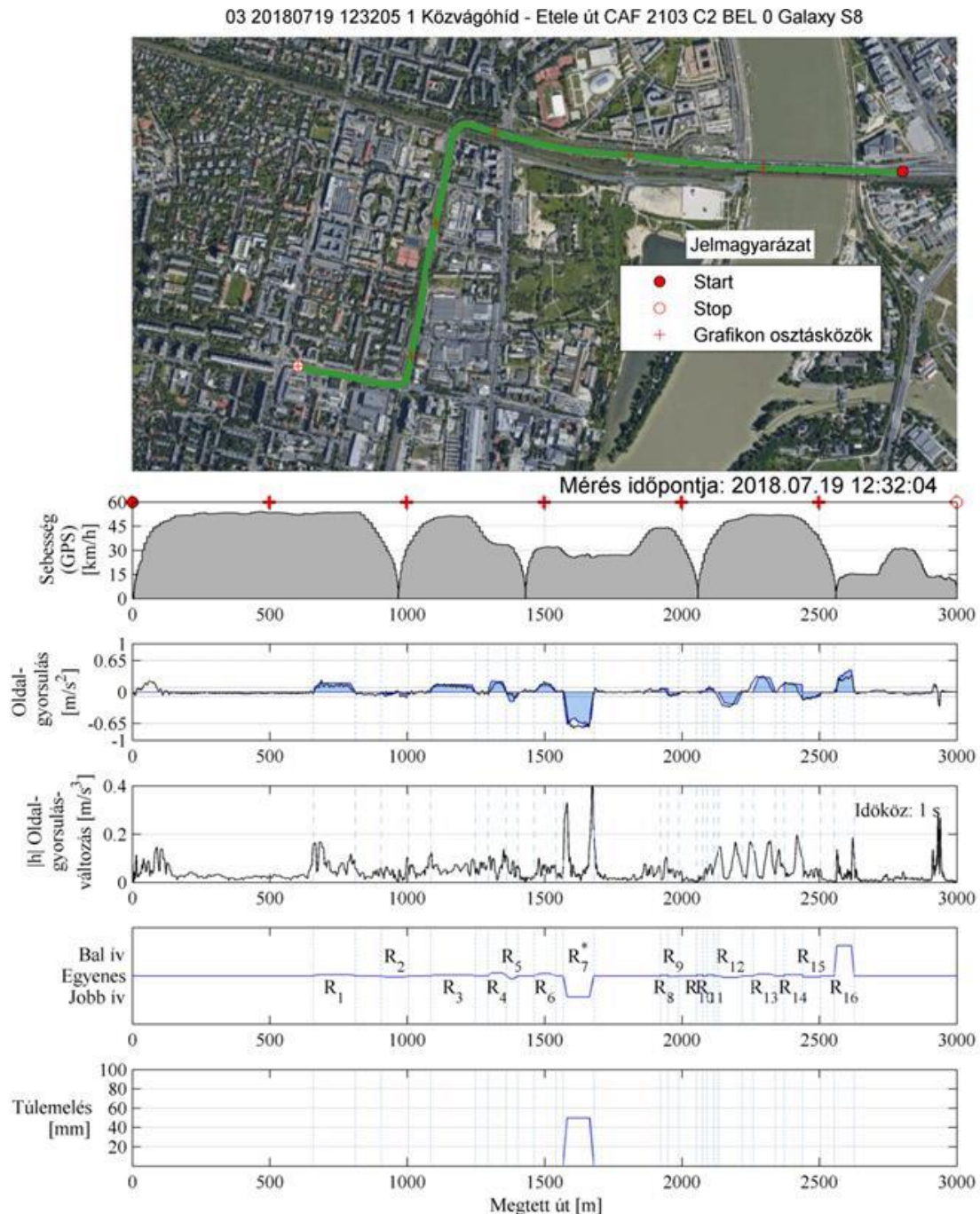
37. ábra: Ívviszonyok jellemzése: a C2 modul bal első ablakán mért kocsiszekrény oldalgyorsulás és a közelítő képletekkel számított gyorsulásadatok összehasonlítása
