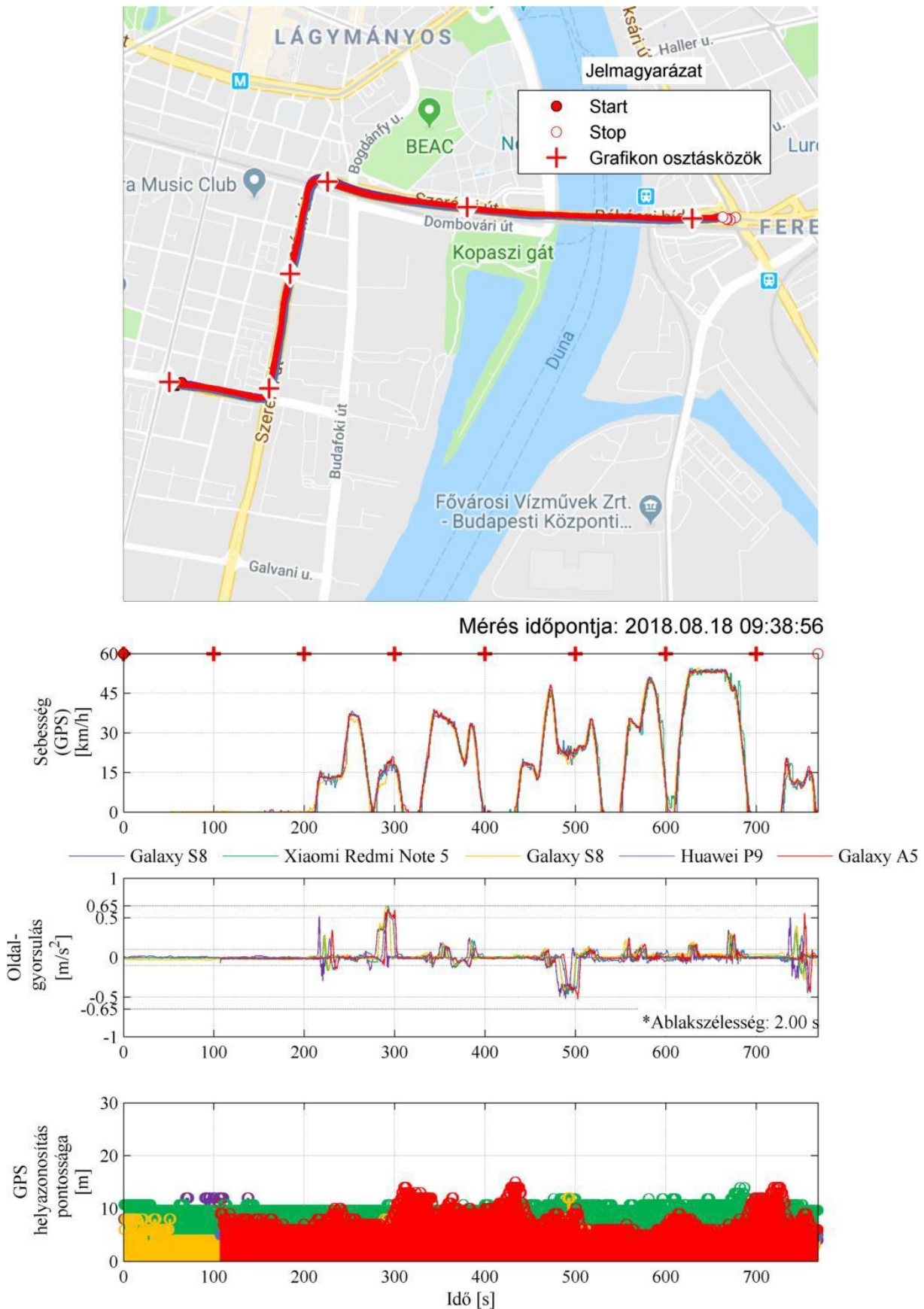
36. ábra: CAF 9 modulok szerelvény vizsgált keresztmetszeteiben rögzített oldalgyorsulás (Etele út/Fehérvári út - Közvágóhíd)
