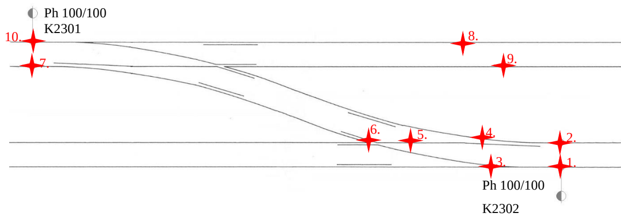
51. ábra: A Clark Ádám téri vonali visszafogás használatból eredő avulási jelenségeinek elhelyezkedése [45]
