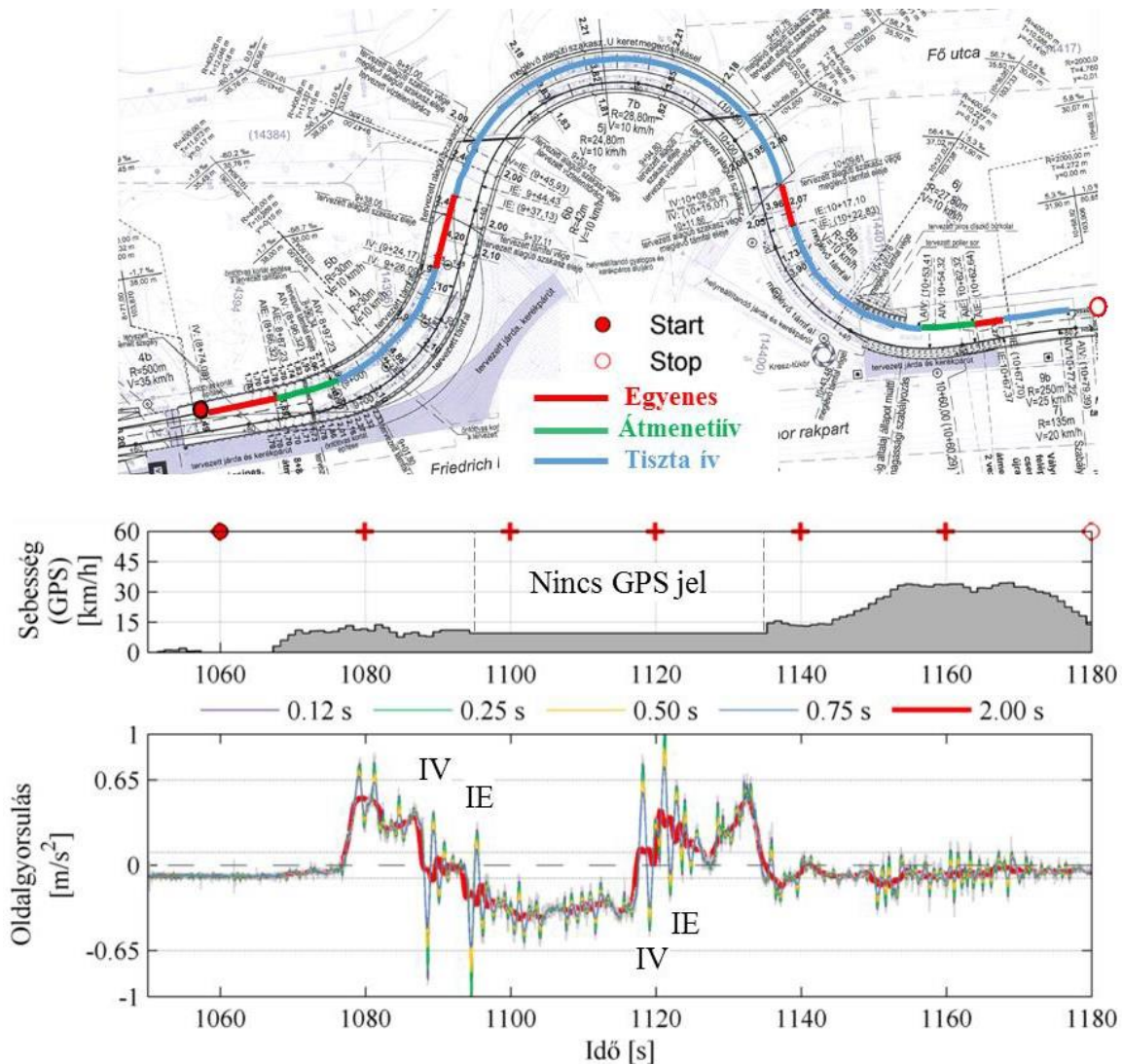
13. ábra: Különböző időablak szélességre meghatározott oldalgyorsulás mozgóátlag vizsgálata a Clark Ádám téri Lánchíd alagútban (Samsung Galaxy A5, CAF 2209 menetirány szerinti első vezetőfülke ablakán mérve a Batthyány tér felé) (konzulensi segítséggel történő kiértékelés)
