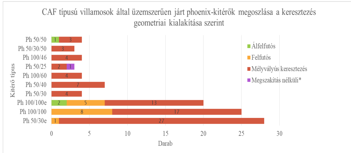
22. ábra: CAF típusú villamosok által járt Phoenix-kitérők megoszlása a keresztezési csúcs geometriai kialakítása szerint 14,15,16
