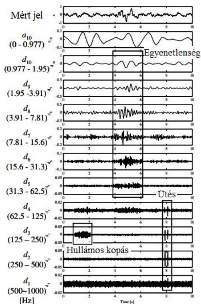
7. ábra: A pályahibák azonosítása különböző frekvenciatartományokban [19]
