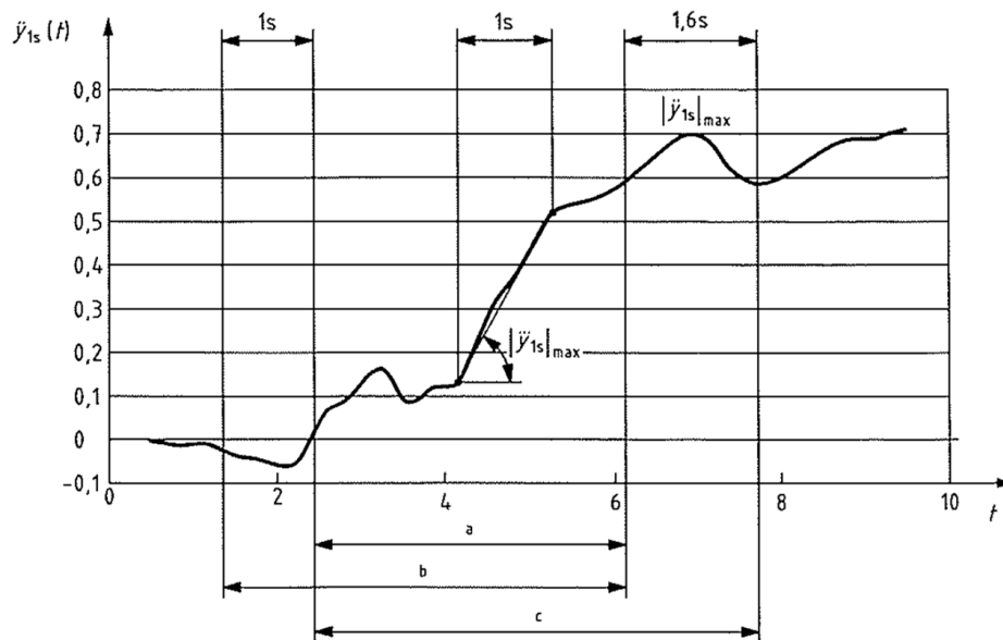
9. ábra: Oldalgyorsulás adatok kiértékelése a P_{CT} módszer szerint [39]
