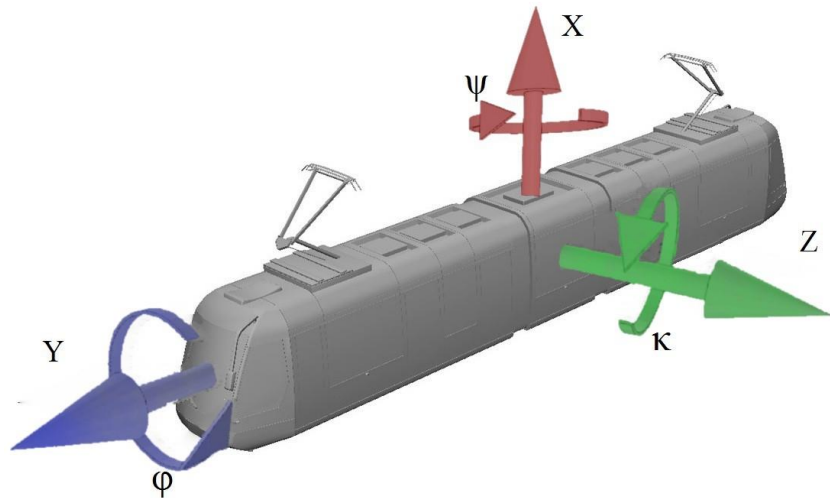
10. ábra: CAFat applikáció mérési tengelyeinek értelmezése és a szabálytalan járműfutás kapcsolata
