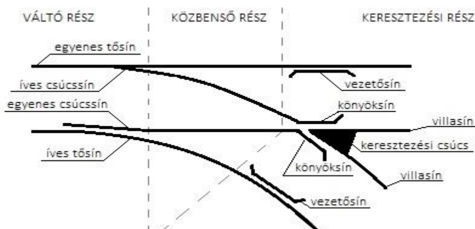
3. ábra: A kitérő szerkezeti egységei
