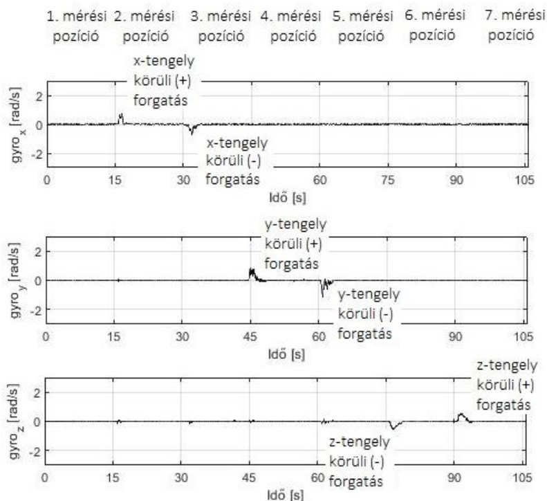
31. ábra: A dőlésmérő kalibráció giroszkóp adatainak ábrázolása (30. ábra szerinti mérési folyamat)
