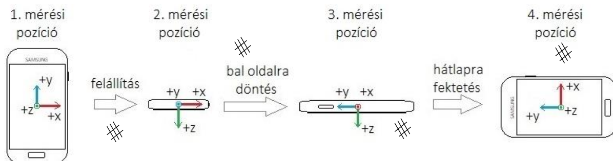
26. ábra: A gyorsulásmérő és a giroszkóp szenzor kalibrálása során vizsgált mérési pozíciók felülnézetben ábrázolva
