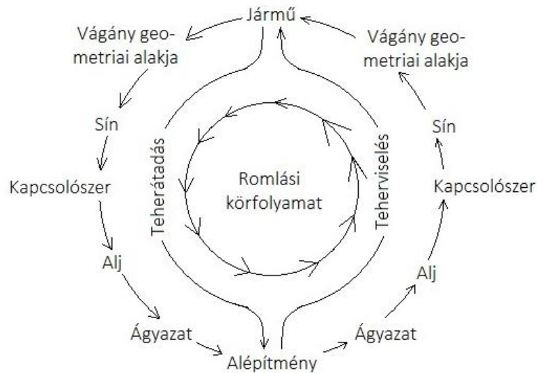
1. ábra: Avulás öngerjesztő romlási körfolyamata [6]
