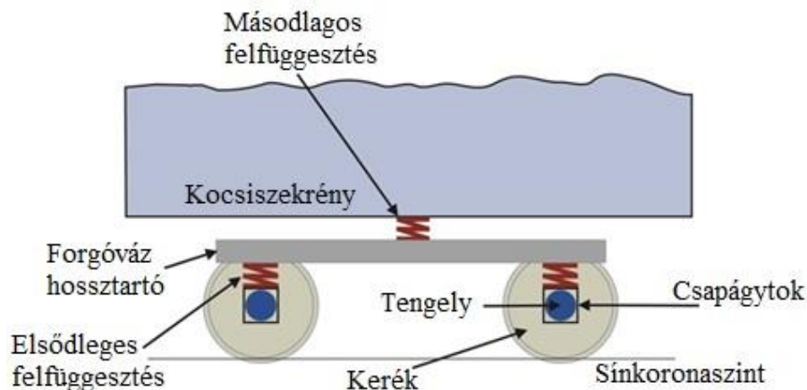
5. ábra: Kéttengelyes, forgóvázvas vasúti jármű egyszerűsített részmodellje
