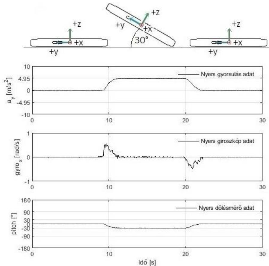
17. ábra: A gyorsulásmérő, giroszkóp és dőlésmérő közötti különbség szemléltetése: 30°-os elforgatás az x-tengely körül
