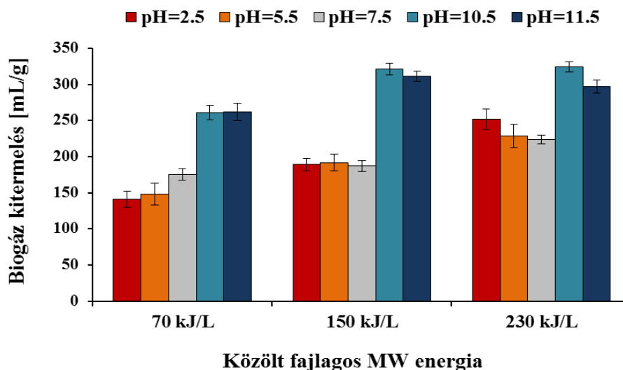
2. ábra. Tejipari iszaphól keletkező biogáz mennyisége (30 napos kumulált térfogatból)
