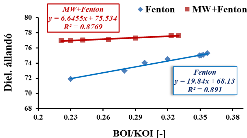
5. ábra. Dielektromos állandó és BOI/ KOI arány kapcsolata tejipari szennyvíznél (Fenton eljárás és MW+Fenton eljárással kezelt mintáknál, 400 MHz frekvencián)
