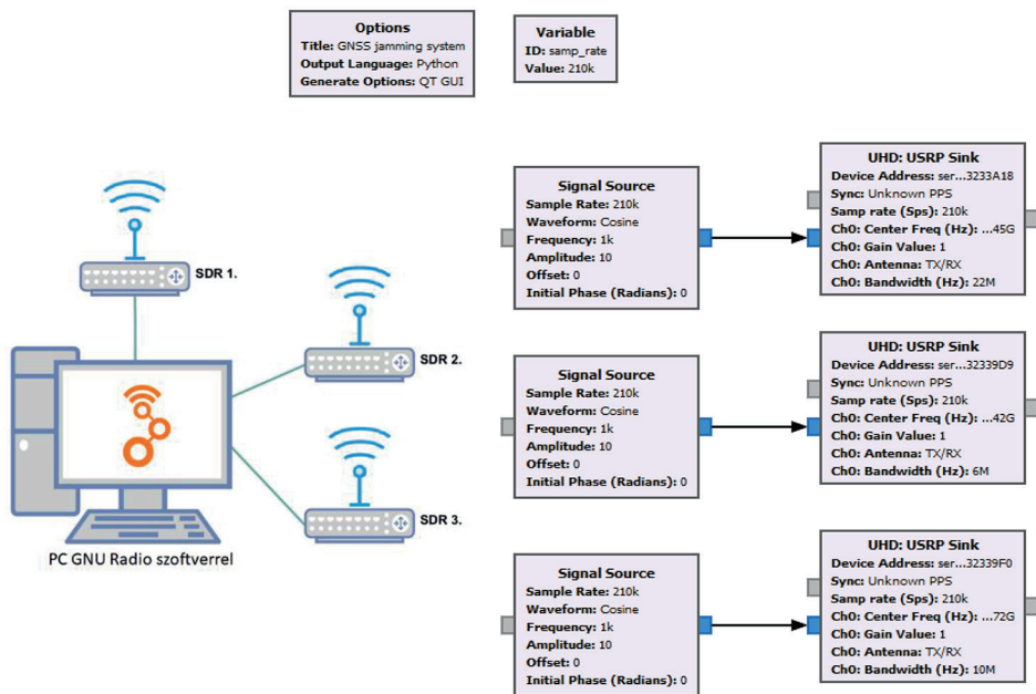
2. ábra Mérés környezete és minta GNU Radio-kód [a szerzők]
