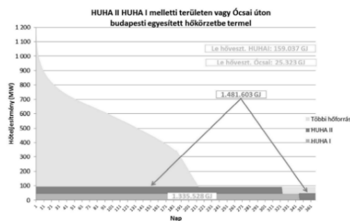
1. ábra: A HUHA 2 tervezett menetrendjének tartamdiagramja [1]
