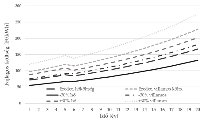
3. ábra: A fajlagos hő- és a villamos költségek alakulása a gázár változásával
