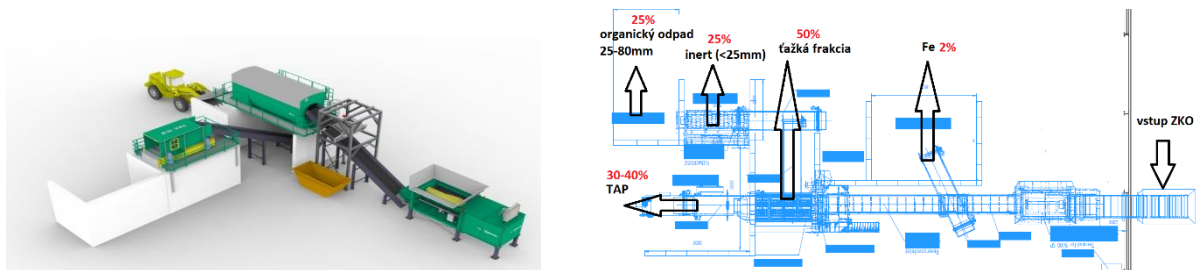
Obr. 5 a 6 Jednoduchá mechanická triediaca linka na ZKO a výstupy zo spracovania
